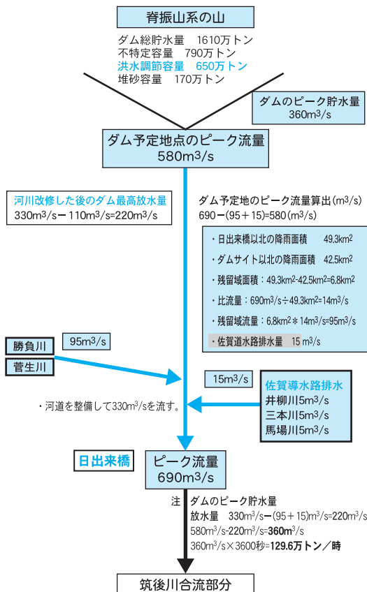
ダム予定地点のピーク流量の数値的考察 (国土交通省案)
