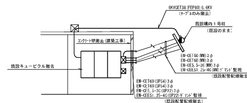
キュービクル周り (現況・撤去前) (A3) S=1/150
