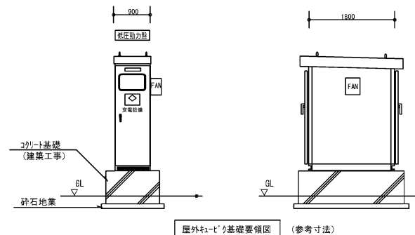
屋外キュービクル基礎要領図 (参考寸法)
