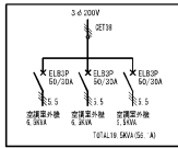
図 3-3 空調機外機接続図
