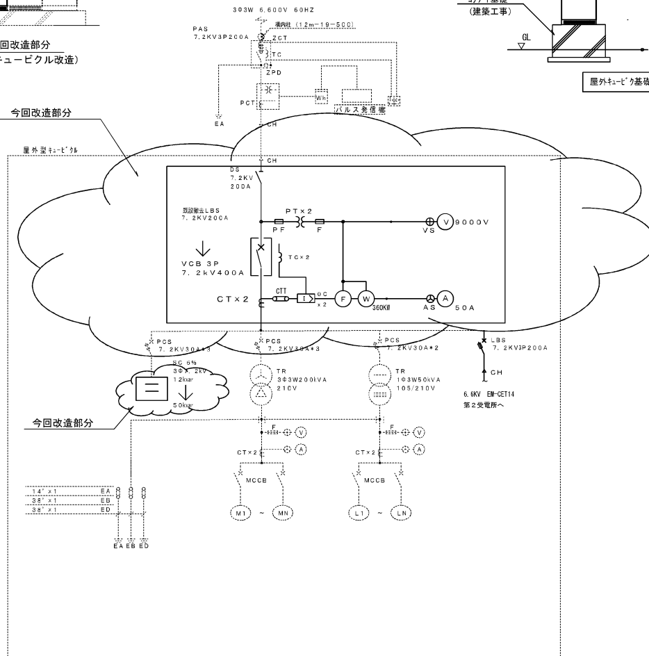
第1受電所 (既設改造)
