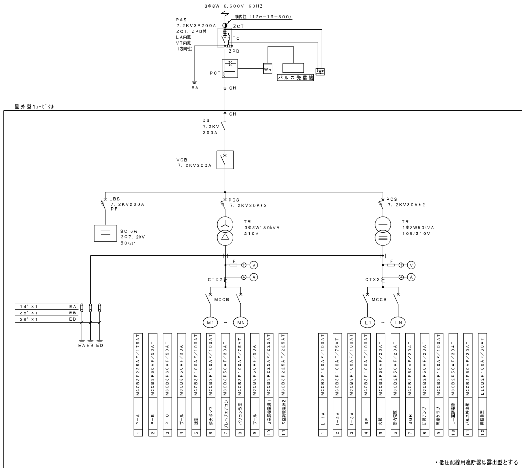
高圧受設備
