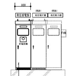
今回改造部分 (既設キュービクル改造)
