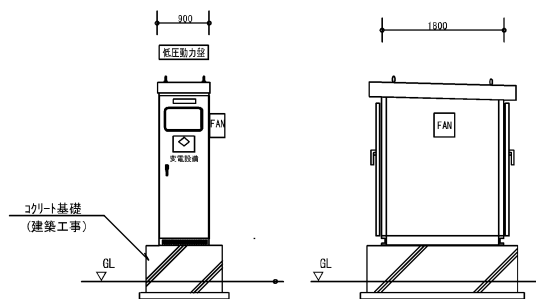
屋外キュービクル基礎要領図 (参考寸法)
