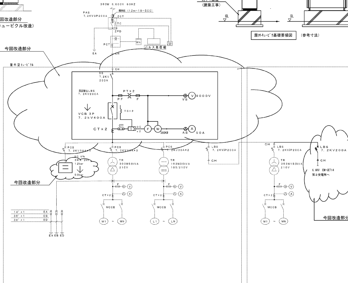
第1受電所 (既設)
