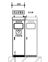
今回改造部分 (既設キュービクル改造)
