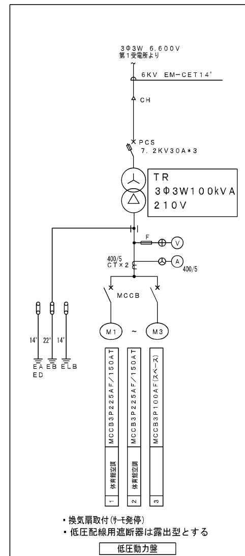
屋外キュービクル1面体
