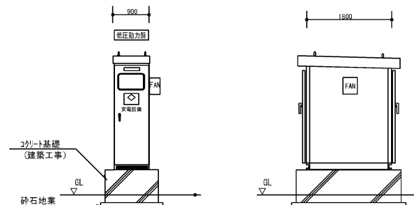
屋外キュービクル基礎要領図 (参考寸法)
