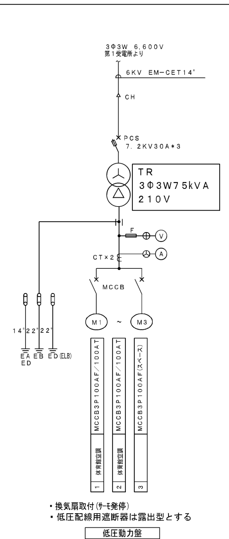
屋外キュービクル1面体
