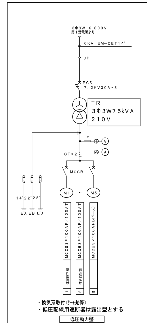
屋外キュービクル1面体
