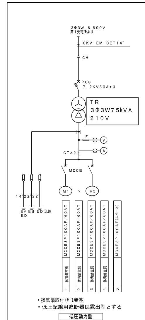
屋外キュービクル1面体 第2受電所（B）タイプ
