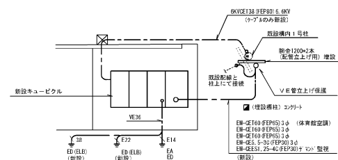
キュービクル周り (改修後) (A3) S=1/150
