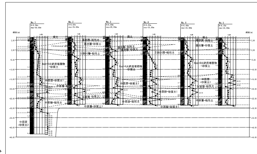
地質推定断面図
