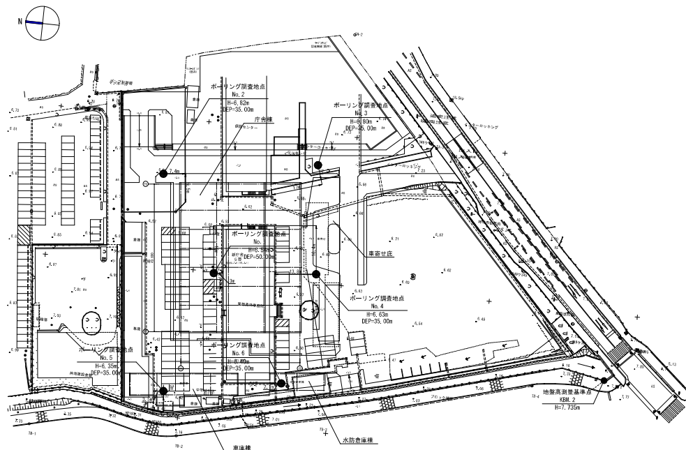
調査位置図 KBM: H=7.735m 設計GL=KBM+165 (H=7.900m)
