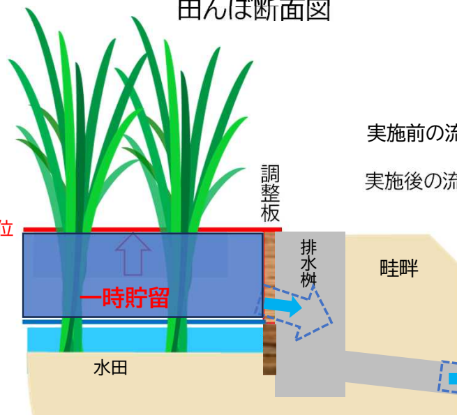
田んぼ断面図
