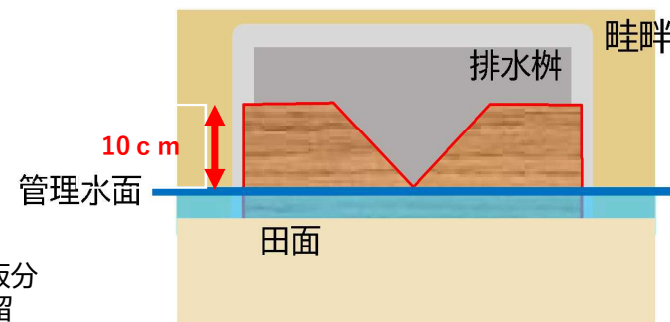
正面図
