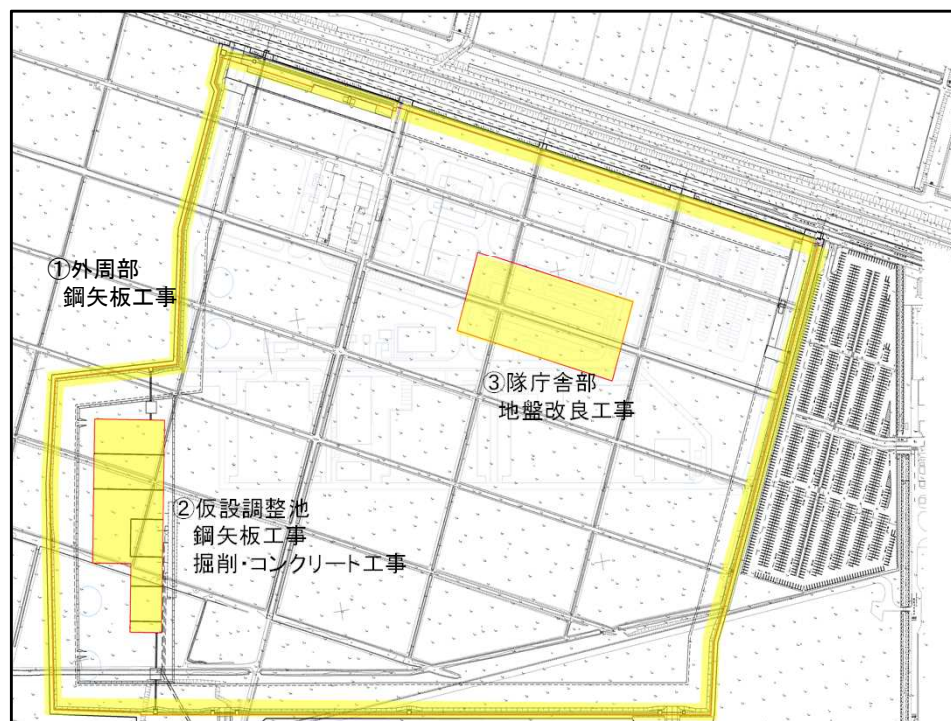
夜間工事 施工範囲平面図
