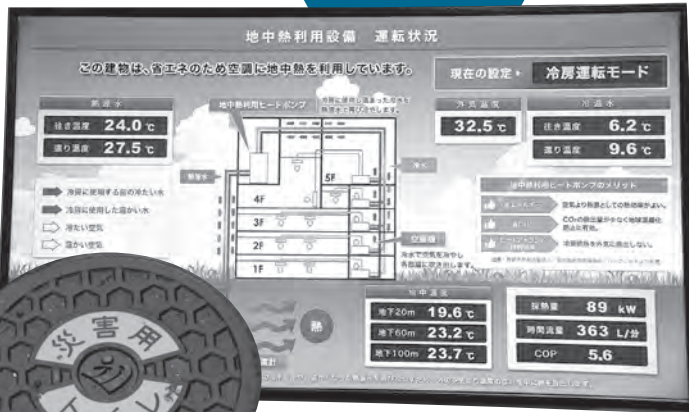
▲地中熱利用設備の運転状況を表示
