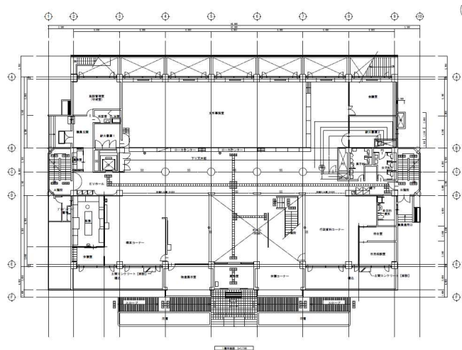
1階平面図 (約 1,000 m 2 )
