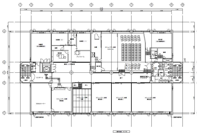
4階平面図 (約 1,000 m 2 )
