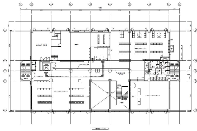
3階平面図 (約 1,000 m 2 )
