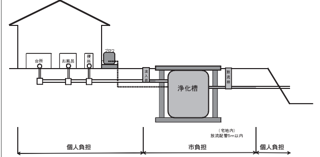
浄化槽設置工事費負担区分図
