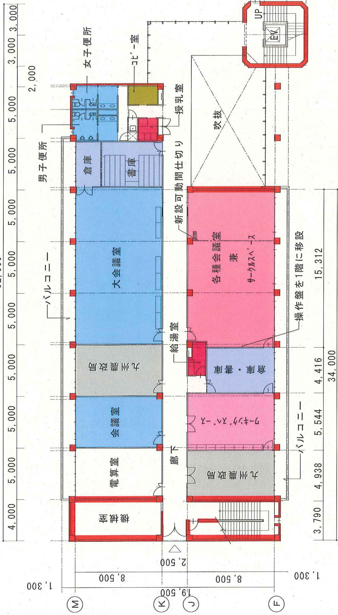
2階平面計画図
